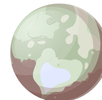
Pluto
