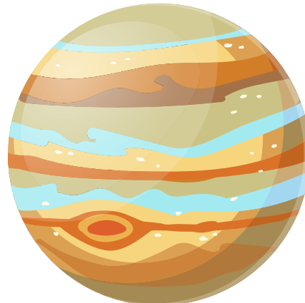
Jupiter
