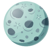
Moon
